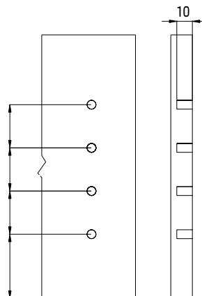
מידות קידוח: קוטר 10 מ"מ, עומק 12 מ"מ
